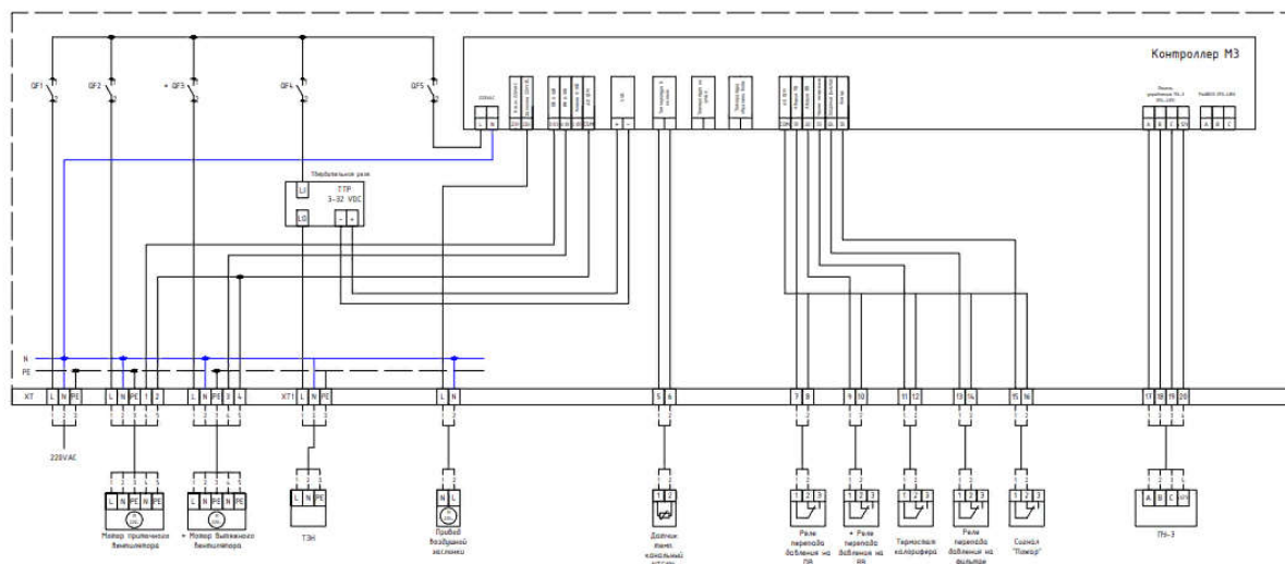
Схема управления с электрическим нагревателем
